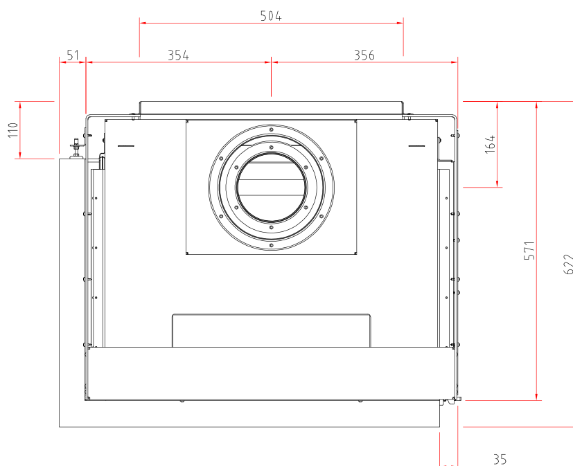
Draufsicht M 1:10
