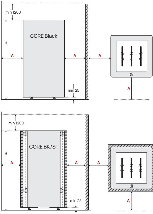
Figur 1. Bastuugns placering
