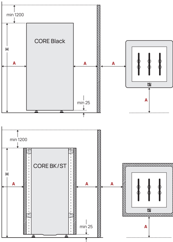
Рисунок 1. Размещение каменки.
